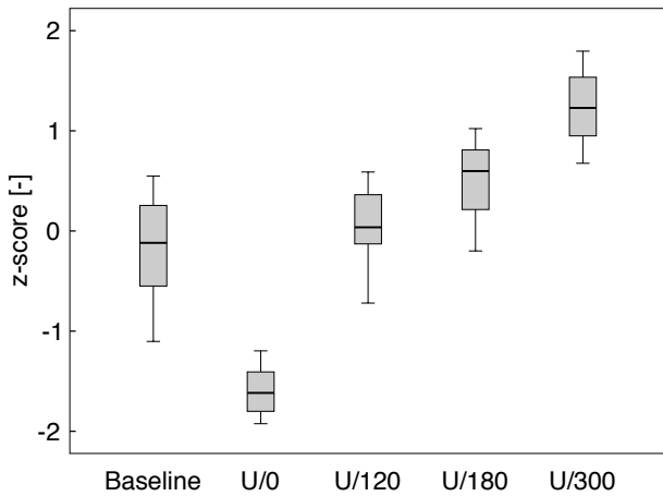
Fig. 10. STA revisions.
