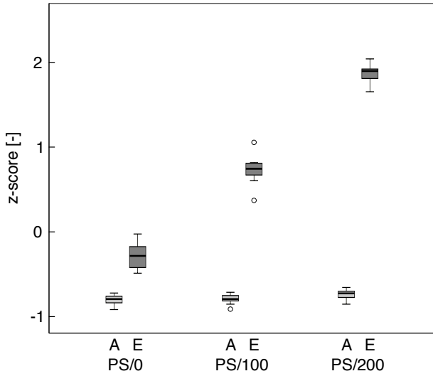
Fig. 5. STA revisions.
